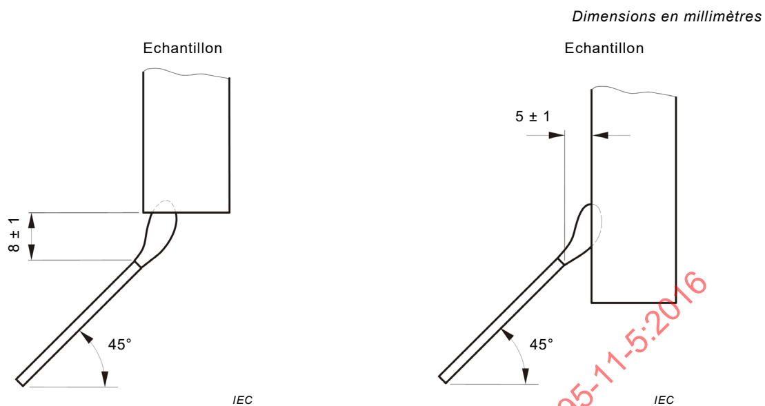
Figure 2a – Position d'essai (exemple horizontal)
