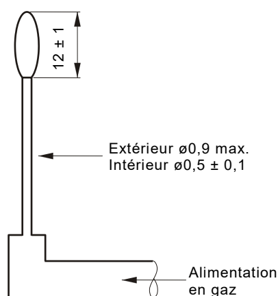
Figure 1 – Brûleur et flamme
