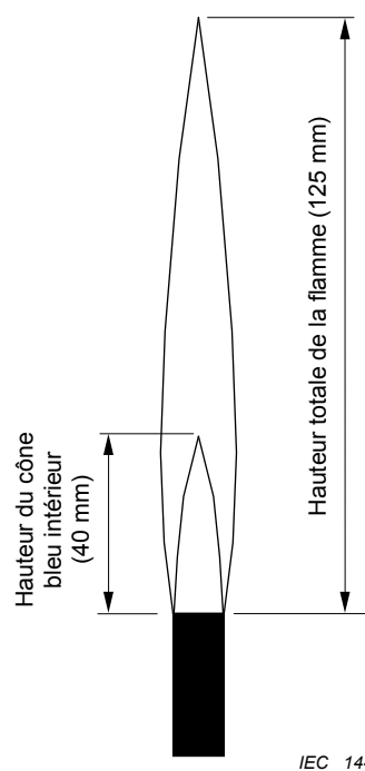
Figure 1 – Dimensions de la flamme
