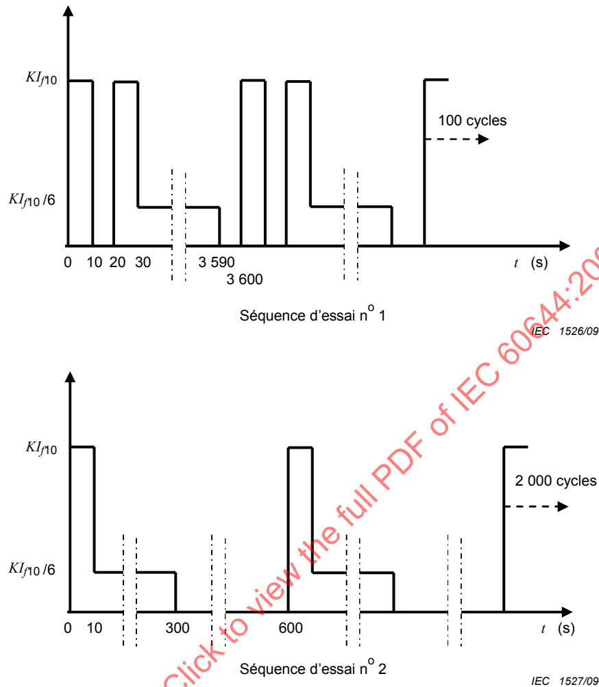
Figure 1 – Diagrammes des séquences d'essai
