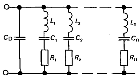
FIG. 1. — Circuit équivalent.
