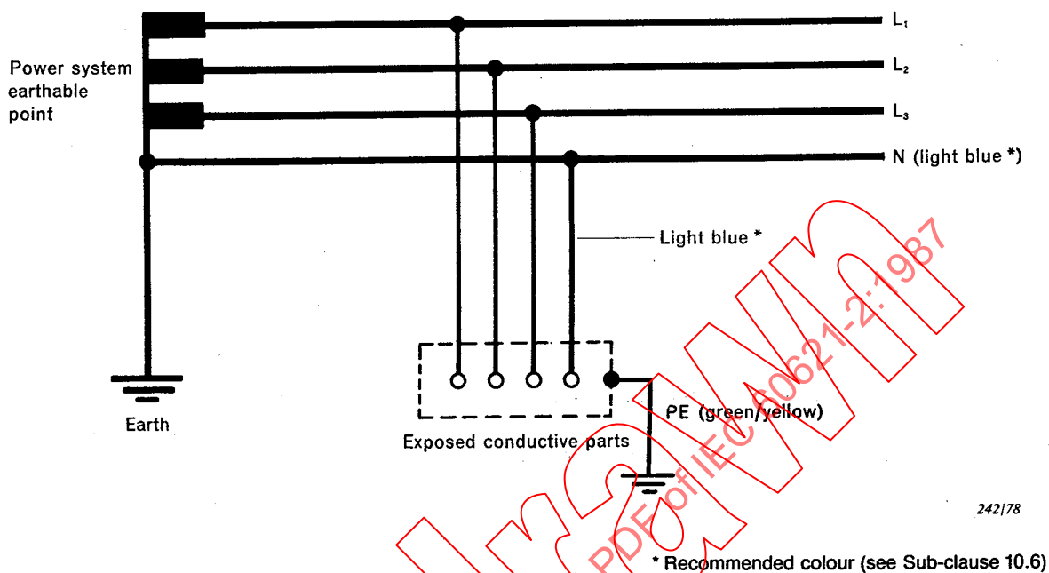
FIG. 10. — Power system TT.
