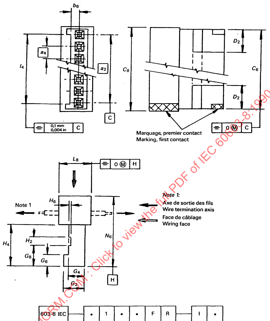
Figure 21 – Fiche pour sorties autodénudantes à sorties perpendiculaires à l'axe d'enfichage, modèle carte à fil (B ou D) Free connector for insulation displacement terminations with terminations perpendicular to the plug-in axis, board-to-wire style (B or D)
