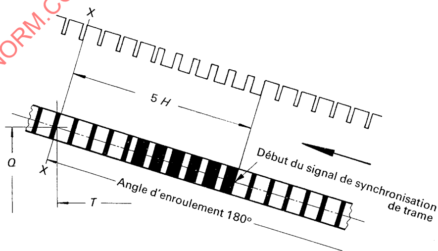
Détail b: Fin de la bande vidéo enregistrée (NTSC).
