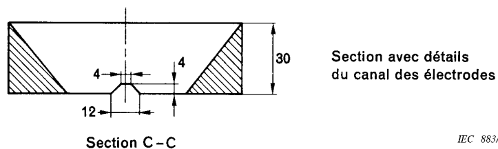
Détail C - Partie supérieure du masque
