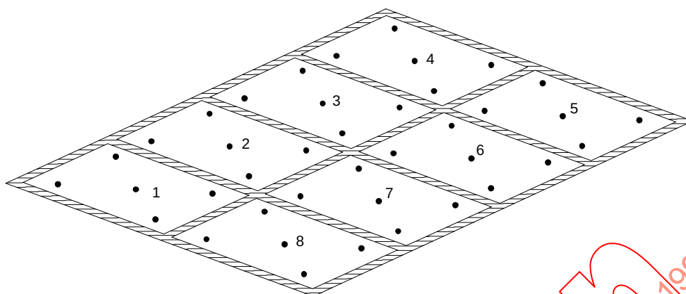
Figure 101a – Position des capteurs de température sur la surface de contact de la zone chauffée d'un DISPOSITIF DE RÉCHAUFFAGE (voir 2.12.101, 50.101 et 50.105)
