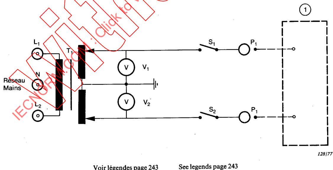
FIG. 11. — Circuit d'alimentation de mesure avec le RÉSEAU D'ALIMENTATION approximativement symétrique par rapport à la terre (voir paragraphe 19.4b)). Measuring supply circuit with the SUPPLY MAINS approximately symmetrical to earth (see Sub-clause 19.4b)).
