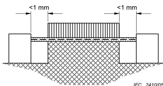
Figure 27 – LIGNE DE FUIITE et DISTANCE DANS L'AIR – Exemple 6
