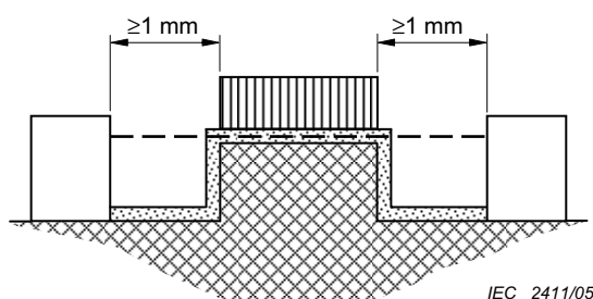
Figure 28 – LIGNE DE FUIITE et DISTANCE DANS L'AIR – Exemple 7
