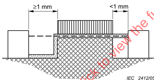
Figure 29 – LIGNE DE FUIITE et DISTANCE DANS L'AIR – Exemple 8
