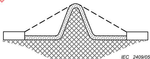
Figure 26 – LIGNE DE FUITE et DISTANCE DANS L'AIR – Exemple 5
