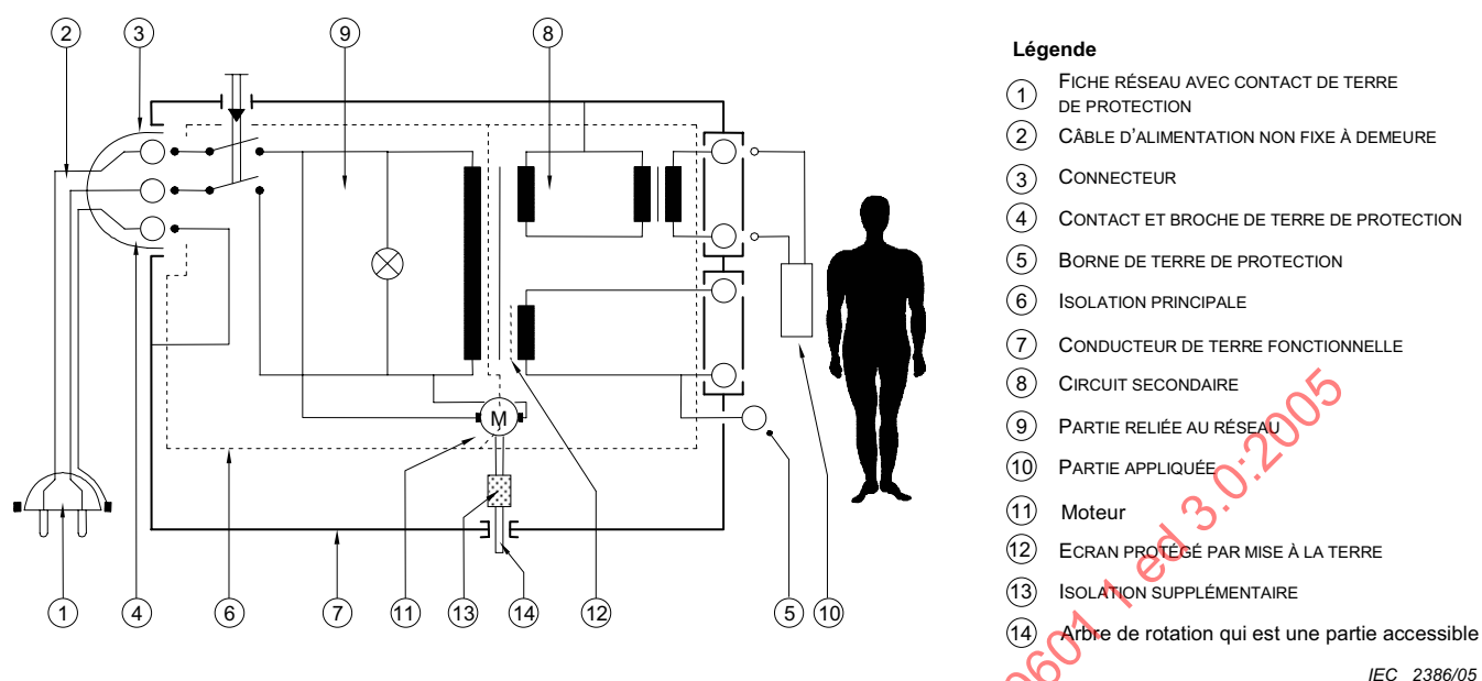
Figure 3 – Exemple d'APPAREIL EM DE CLASSE I (voir définitions)
