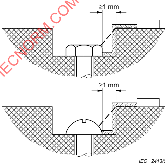
Figure 30 – LIGNE DE FUIITE et DISTANCE DANS L'AIR – Exemple 9
