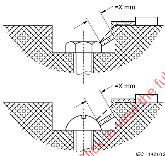
Figure 31 – LIGNE DE FUIITE et DISTANCE DANS L'AIR – Exemple 10
