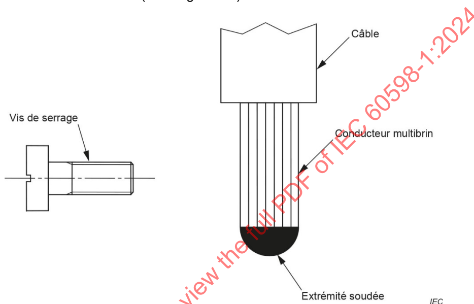
Figure 36 – Exemple de degré d'étamage admis
