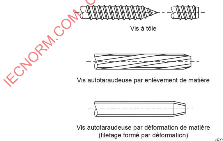
Figure 32 – Exemples de vis à tôle et de vis autotaraudeuses par enlèvement ou déformation de matière
