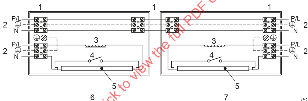
b) "ligne traversante" avec câblage interne séparé électriquement de la ligne traversante
