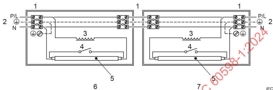
a) "ligne traversante" avec câblage interne raccordé électriquement à la ligne traversante
