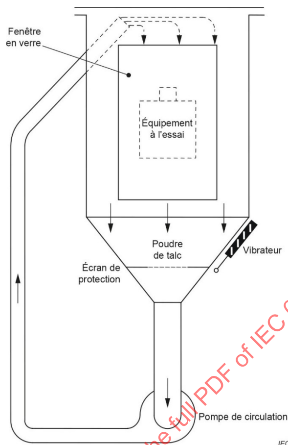
Figure 40 – Appareil pour la vérification de la protection contre les poussières
