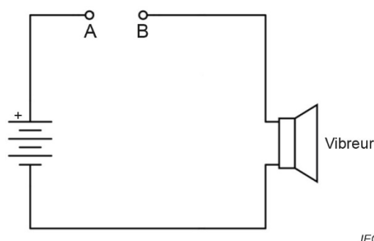
Figure 37 – Circuit pour vérifier le contact électrique entre un socle de prise de courant et une fiche
