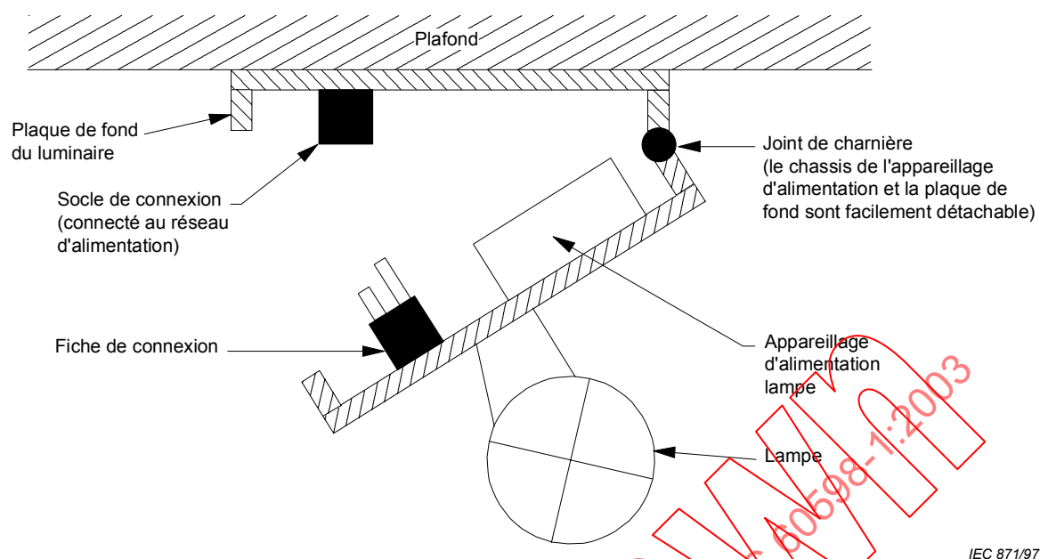
Figure 31 – Système de contact électromagnétique avec connexion fiche socle
