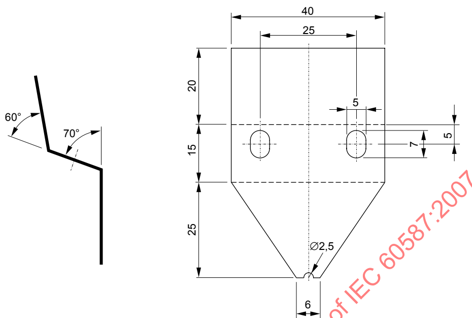
Figure 4 – Électrode supérieure en acier inoxydable de 0,5 mm d'épaisseur
