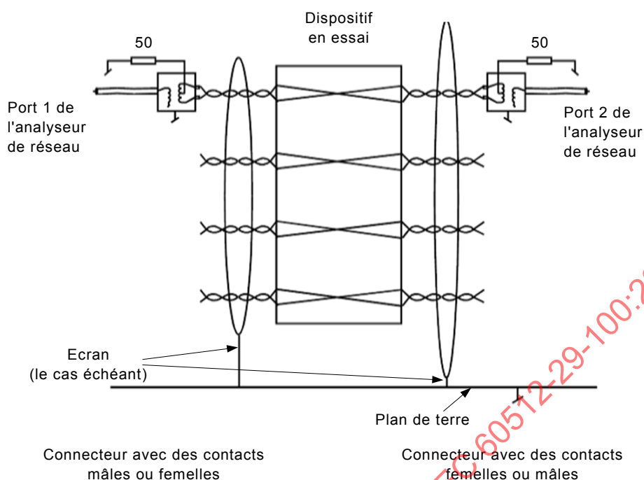
Figure 15 – Montage de mesure
