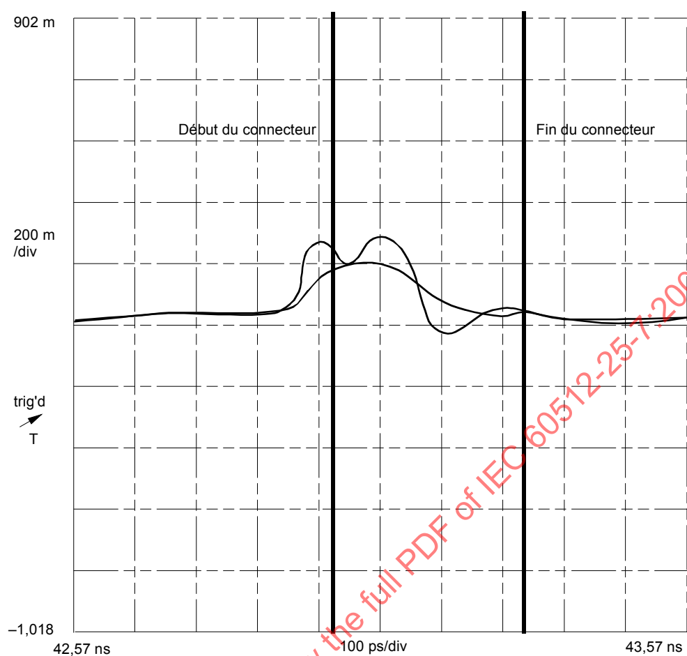
Figure A.2 – Exemple de sortie TDR, 2 courbes (temps de montée différents) et points de l'éprouvette de début et de fin
