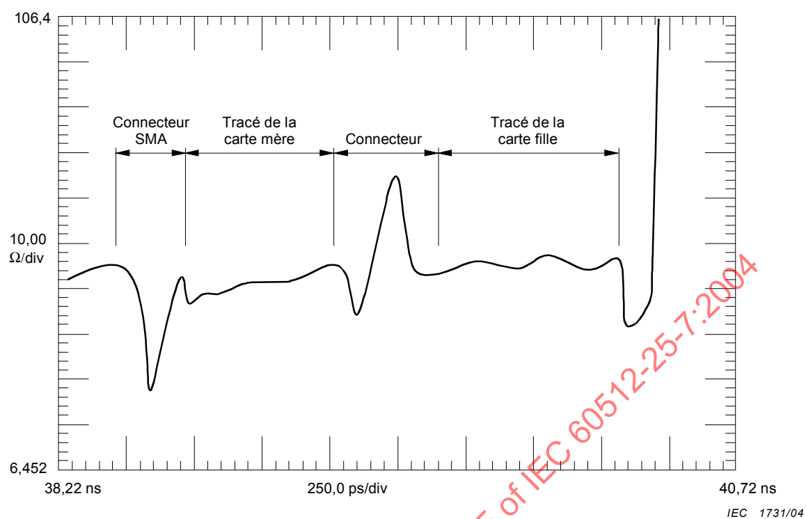
Figure D.1 – Exemple d'un profil d'impédance d'un connecteur utilisant un temps de montée du système de mesure de 35 ps
