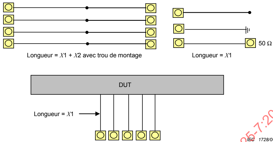
Figure C.1 – Fixation d'essai type carte mère
