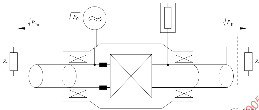
Figure 5 – Schéma du circuit de mesure
