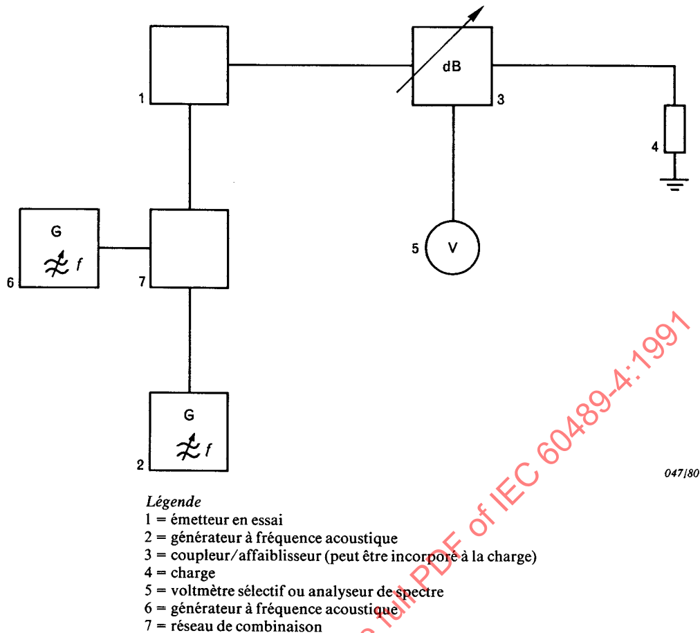
FIG. 9. — Montage de mesure des caractéristiques de l'émetteur.
