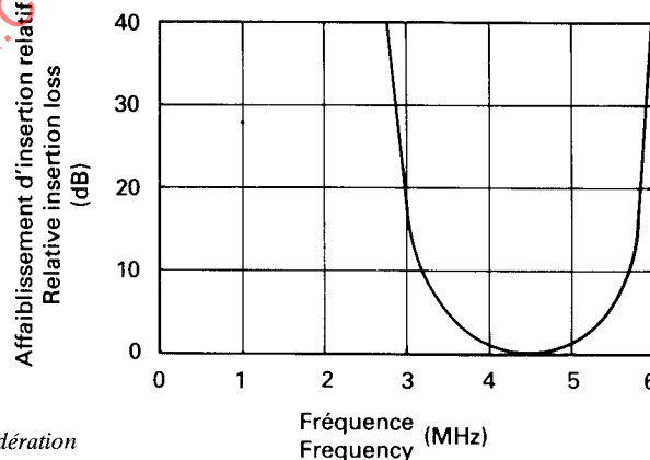
FIG. 4. — Réseau de pondération pour la mesure du bruit dans le canal de chrominance (voir la référence 5). Weighting network for random noise measurement in the chrominance channel (see reference 5).
