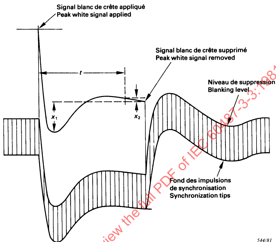
FIG. 5. — Distorsion des signaux de longue durée — aspect typique de la figure obtenue à l'oscilloscope. Long-time waveform distortion — typical oscilloscope display.
