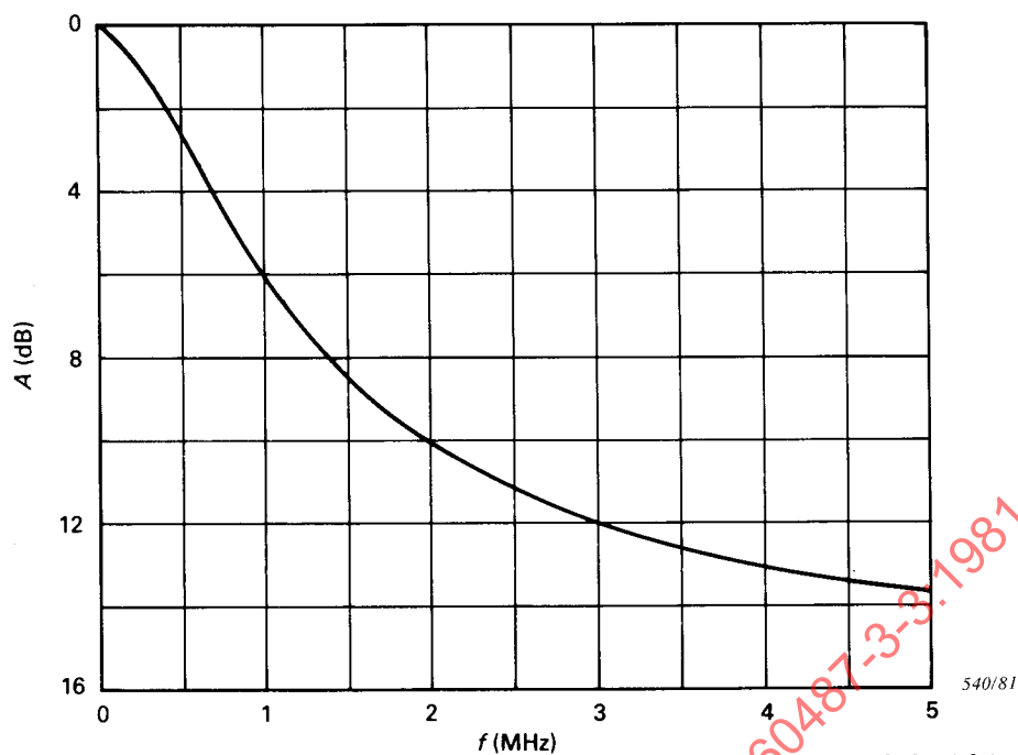
Caractéristiques de pondération unifiée
