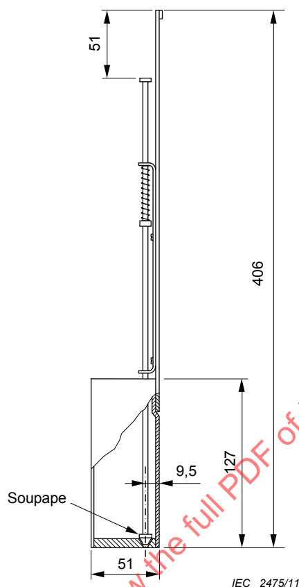
Figure 2 – Écrémoir
