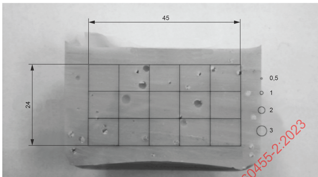
Figure 2 – Position de la grille d'examen sur l'éprouvette
