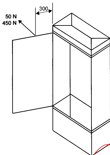
Figure 7 – Dessin pour l'essai de la vérification de la tenue mécanique des portes
