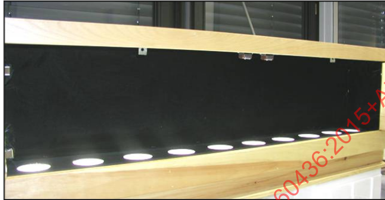
Figure Q.1 – Exemple de boîte lumineuse d'évaluation
