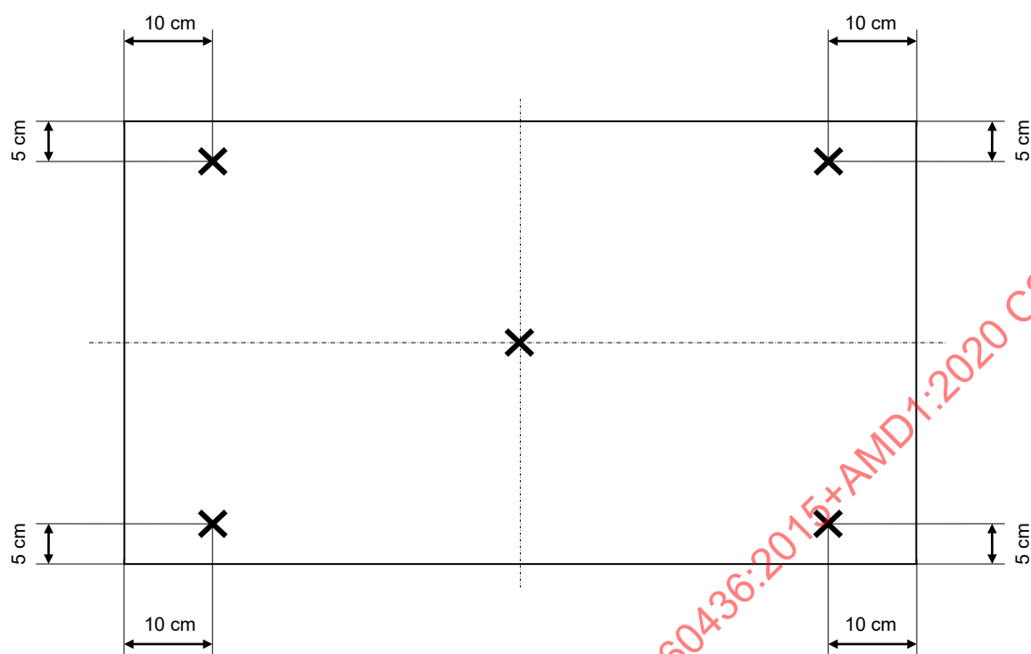
Figure G.1 – Emplacement du thermocouple sur les clayettes supérieures, intermédiaires et inférieures
