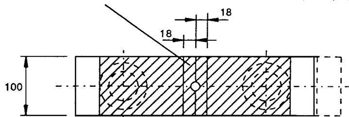
Pièces polaires pour des échantillons de section circulaire (exemple)
