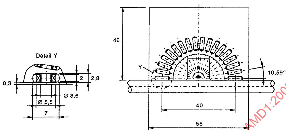
Figure 5e – Système de bobines séparées constituant un potentiomètre de Rogowski-Chattock pour la mesure de I
