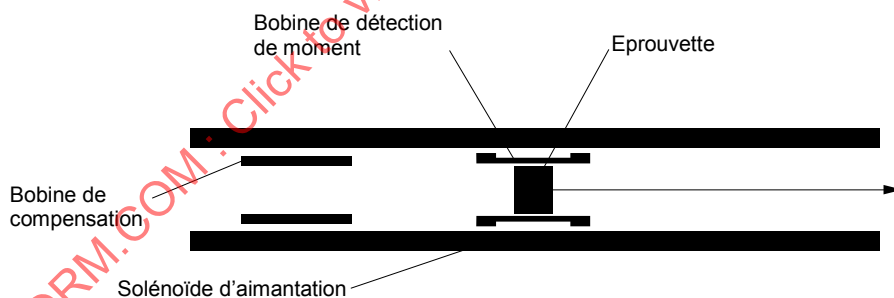
Figure 2 – Système de bobines pour la détermination du moment du dipôle magnétique
