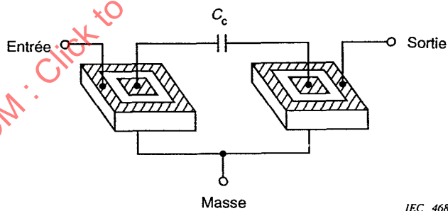
Figure 6 – Filtres associés en cascade
