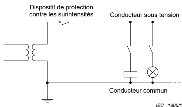
Figure 557.4 – Configuration d'un circuit auxiliaire
