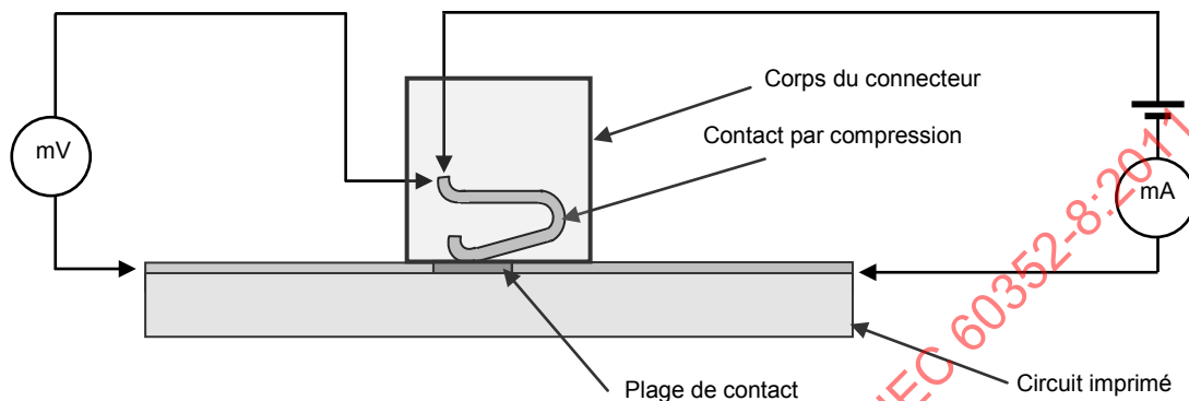
Figure 1 – Disposition du câblage pour l'essai de résistance de contact
