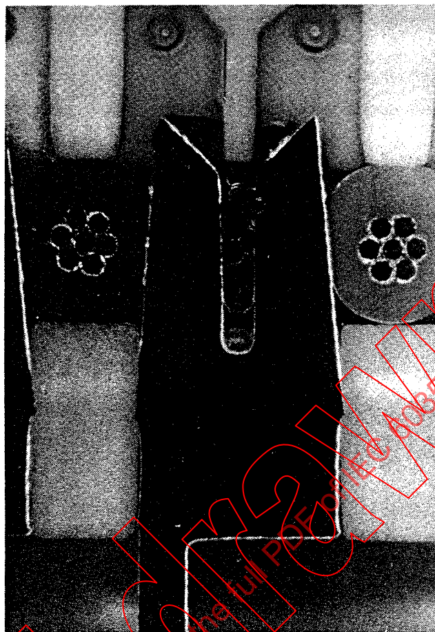
Figure 8 – Connexion CAD non accessible avec un conducteur divisé
