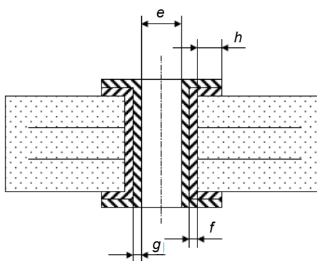
Figure 1 – Trou métallisé
