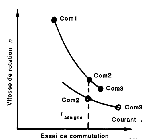
Figure 1c – Moteur de véhicule thermoélectrique
