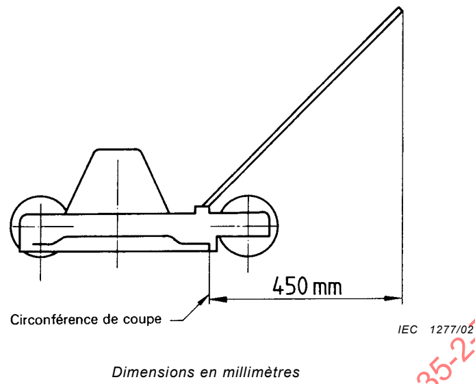
Figure 105 – Longueur du mancheron
