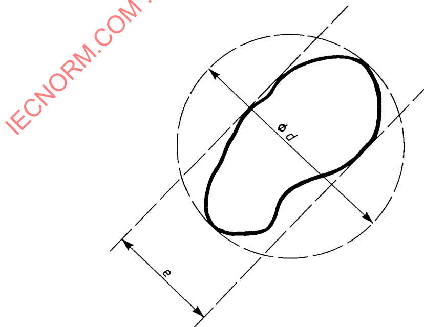
Figure AA.1 – Détermination de l'ouverture nominale
