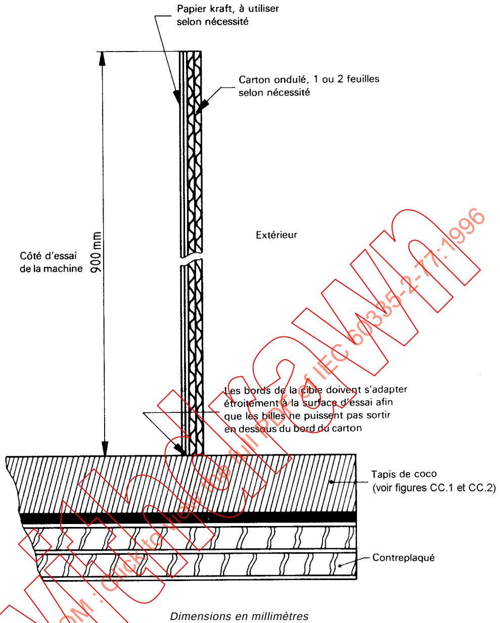
Figure BB.4 – Paroi et support des enceintes d'essai
