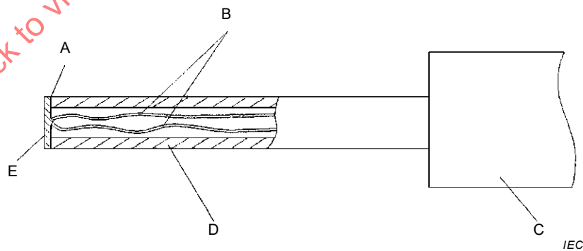
Figure 102 – Identification des surfaces pour la mesure de température
