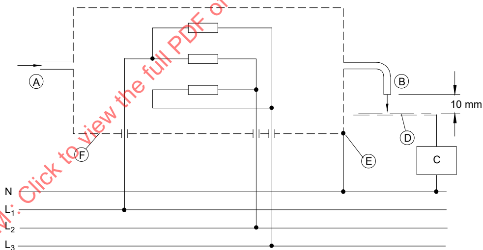
Figure 101 – Schéma pour la mesure du courant de fuite des chauffe-eau à éléments nus monophasés
