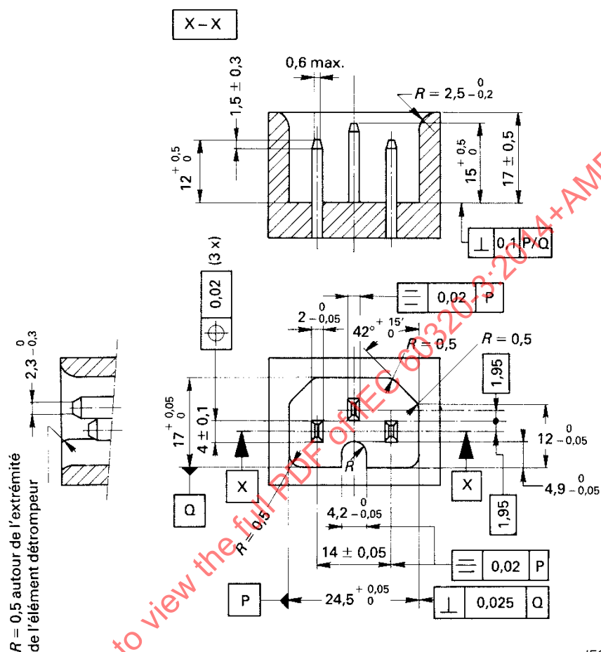
Figure 15 – Calibre "N'ENTRE PAS" pour prises mobiles selon les conformément aux feuilles de norme C13 et C17
