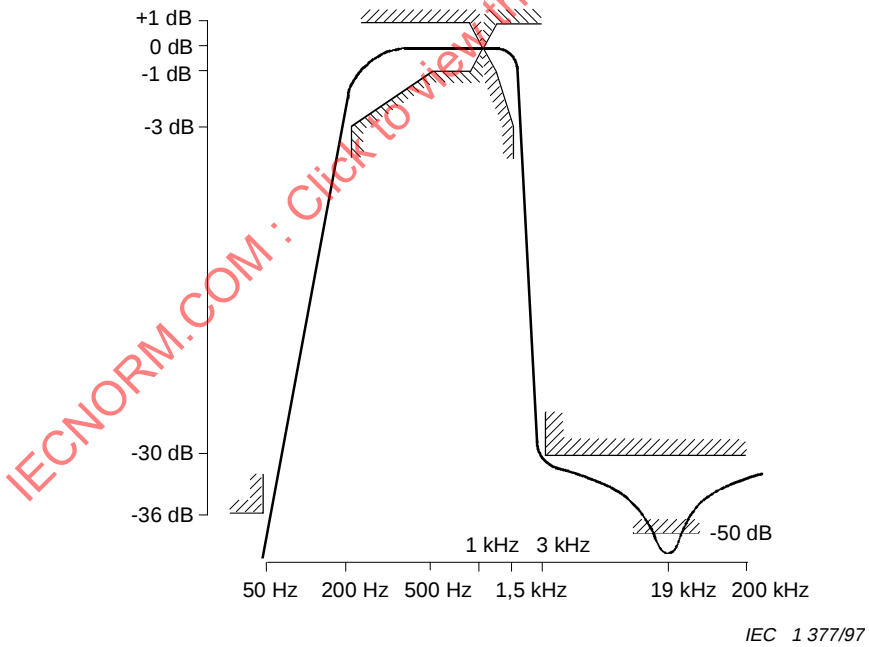
Figure 3 – Limites de la réponse en fréquence du filtre passe-bande 200 Hz à 1,5 kHz
