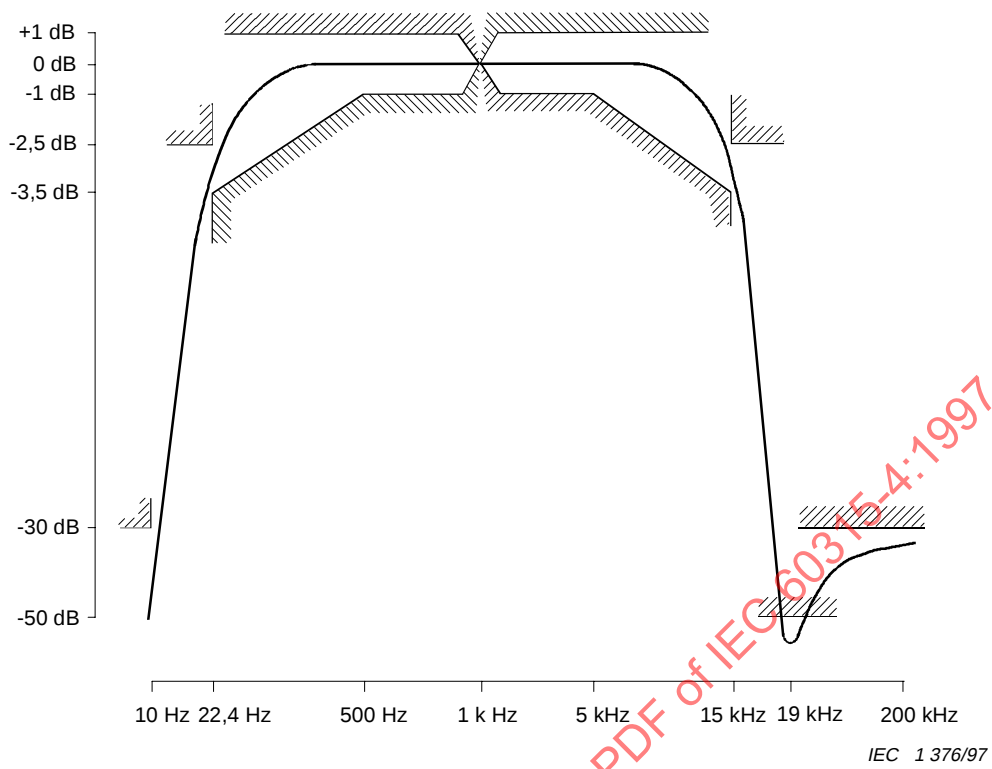
Figure 2 – Limites de la réponse en fréquence du filtre passe-bande 22,4 Hz à 15 kHz
