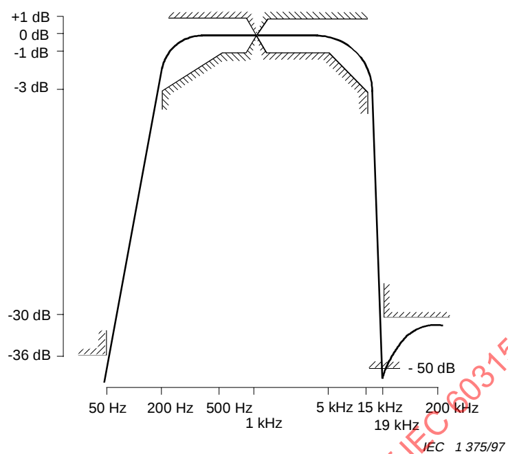
Figure 1 – Limites de la réponse en fréquence du filtre passe-bande 200 Hz à 15 kHz
