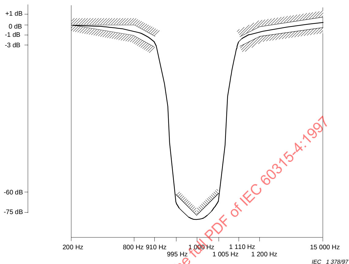
Figure 4 – Limites de la réponse en fréquence du filtre à élimination de bande à 1 kHz
