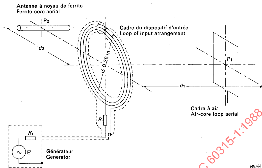
FIG. 8. — Petit cadre blindé (ø 0,25 m) (voir paragraphe 22.2). Small screened loop (ø 0.25 m) (see Sub-clause 22.2).
