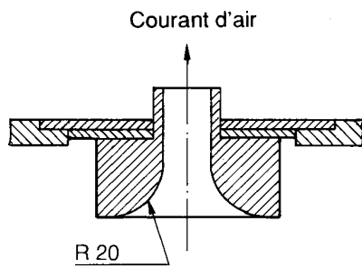
Adaptateur pour la connexion des aspirateurs à conduit d'aspiration
