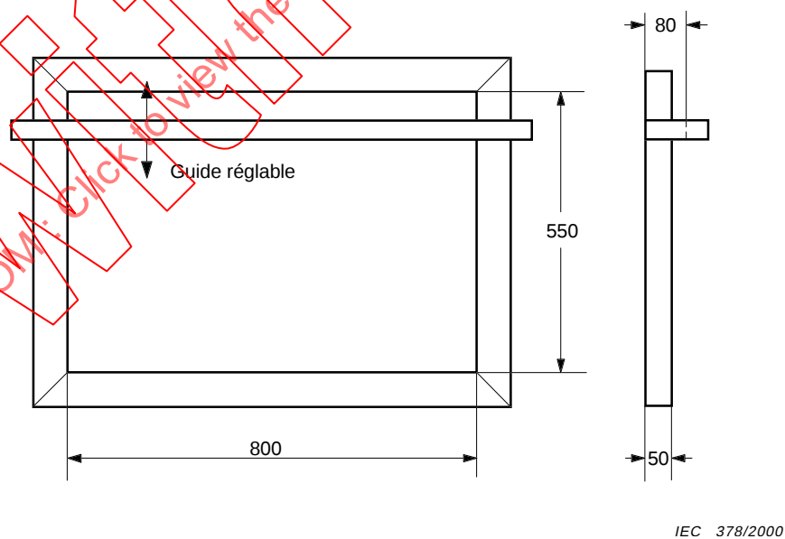
Figure 10b – Cadre pour coussin d'essai
