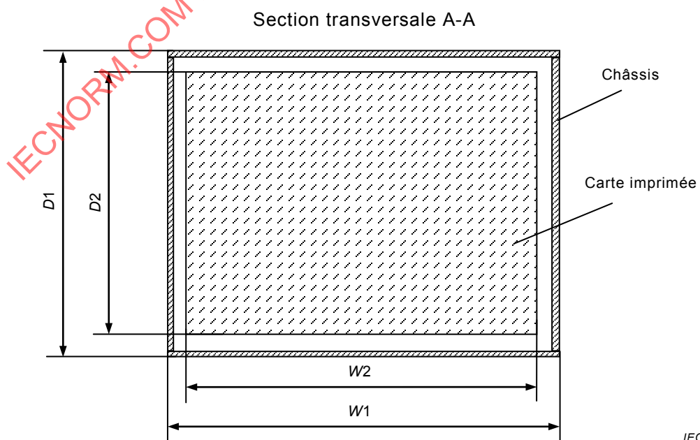
Figure A.2 – Dimensions de la carte imprimée
