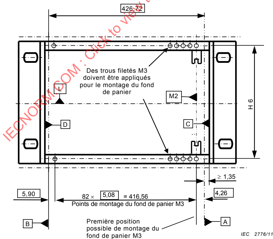
Figure 5 – Dimensions des bacs, vue de derrière
