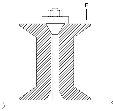
Figure 3 – Porte-bobine (détail de la figure 2)
