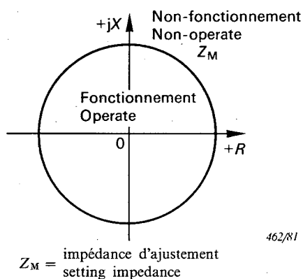
FIG. 1a. — Caractéristique circulaire. Circular characteristic.
