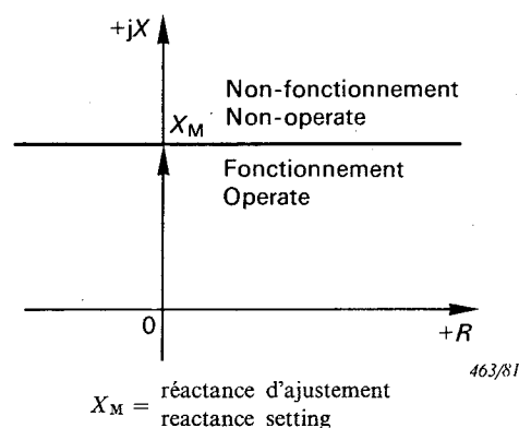
FIG. 1b. — Caractéristique de réactance. Reactance characteristic.
