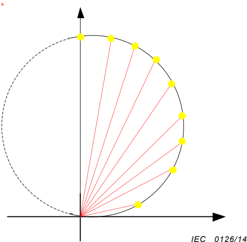
Figure 15 – Caractéristique "MHO" montrant neuf points d'essai
