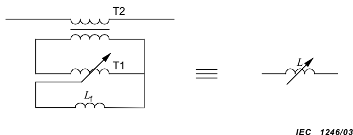
Figure 3 – Montage pour réaliser la bobine d'inductance variable L de la Figure 2
