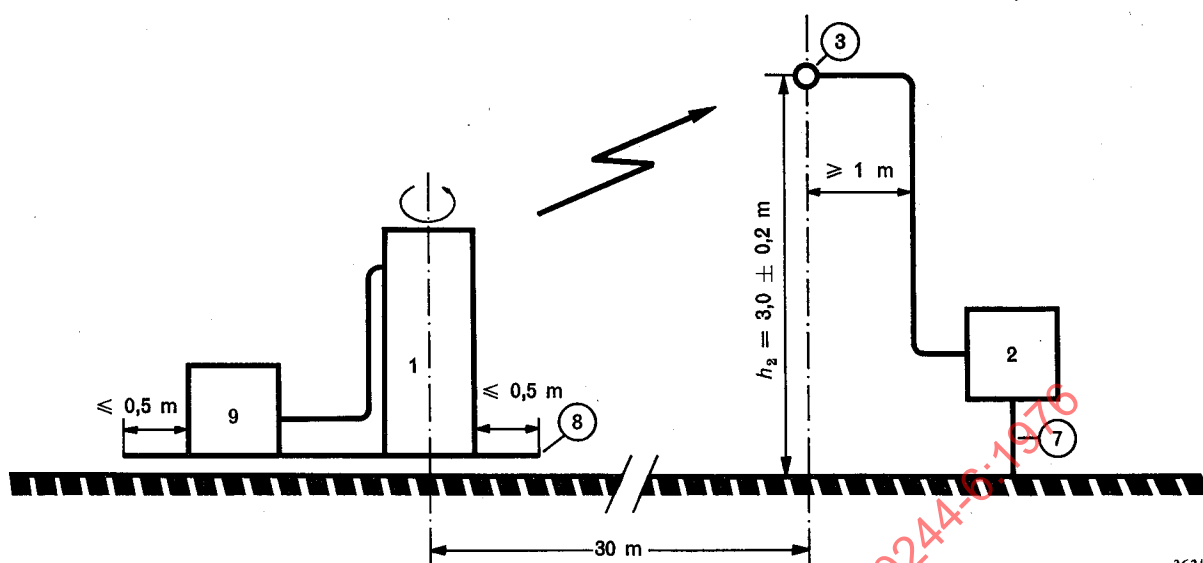
FIG. 3a. — Mesure de rayonnement. Radiation measurement.
