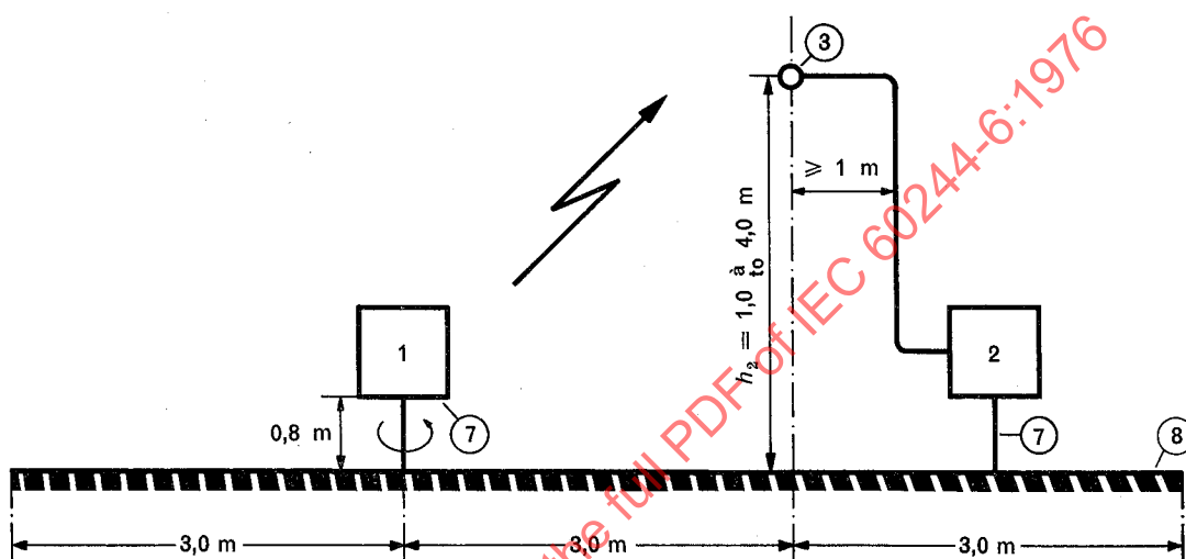
FIG. 2a. — Mesure de rayonnement. Radiation measurement.
