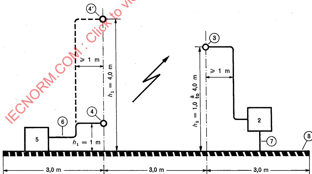
FIG. 2b. — Etalonnage du lieu d'essai et méthode de substitution. Calibration of the test site and substitution method.
