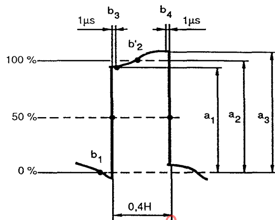
Figure 5i – Signal de barre de luminance de durée ligne Displayed line-time bar signal
