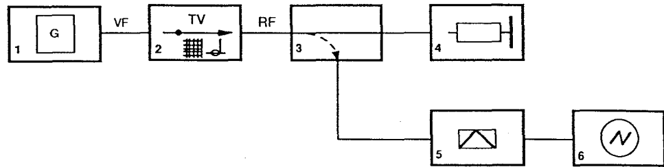
Figure 2a – Montage de mesure pour déterminer la stabilité et les niveaux, des signaux caractéristiques et de l'écrêteur de blanc Measuring arrangement for setting white clipper and characteristic levels and for stability measurement
