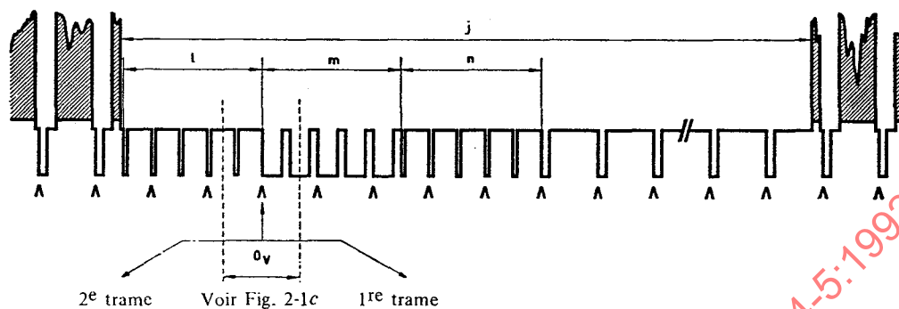
FIGURE 2-1a – Signal au début de chaque 1 re trame
