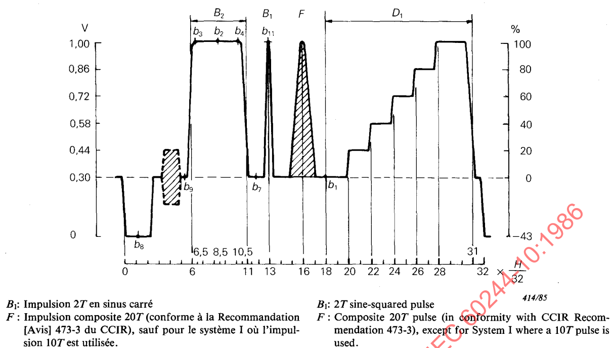
FIG. 1. – Signal d'essai I pour les systèmes à 625 lignes.
