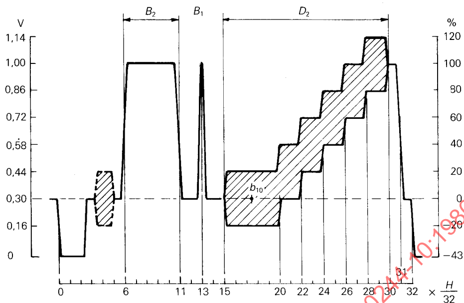
FIG. 3. - Signal d'essai III pour les systèmes à 625 lignes. Test signal III for 625-line systems.
