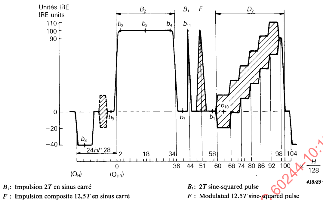
FIG. 5. – Signal d'essai V pour les systèmes à 525 lignes.
