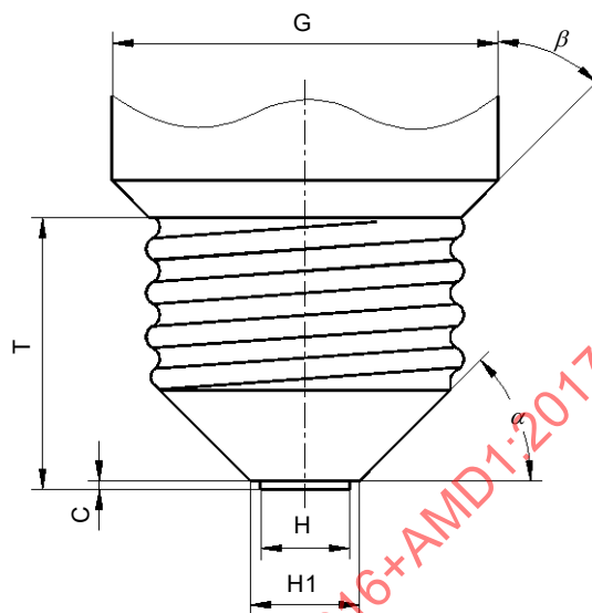
Figure 5b – Culot d'essai E40
