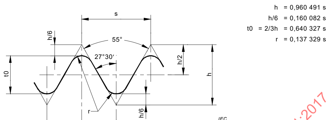
Profil de base a
