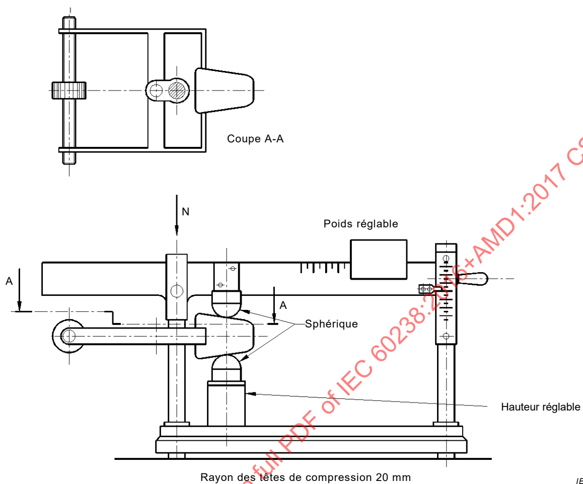
Figure 9 – Appareil pour la résistance à la compression
