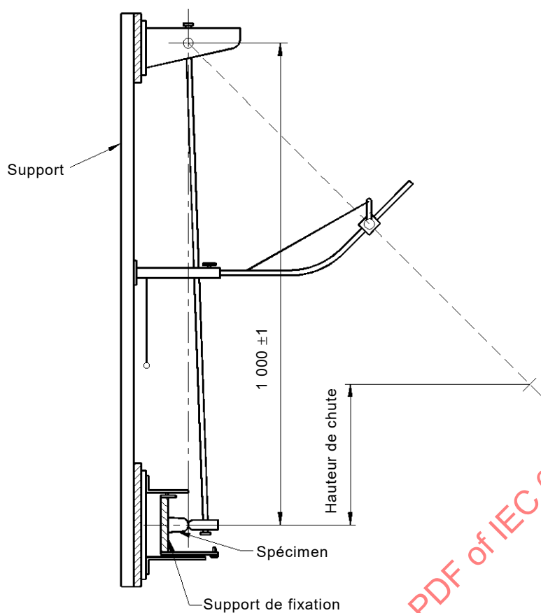
Figure 8a – Appareil pour l'essai de choc
