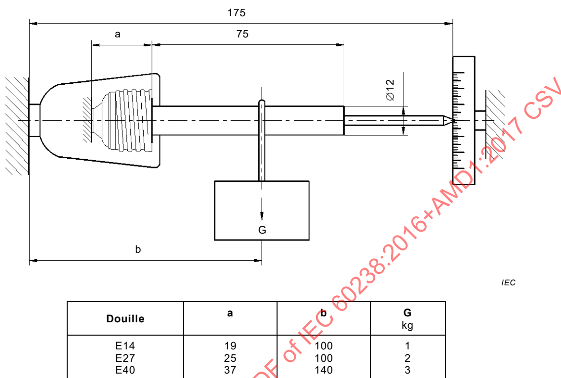
Figure 12 – Appareil pour la résistance à la flexion
