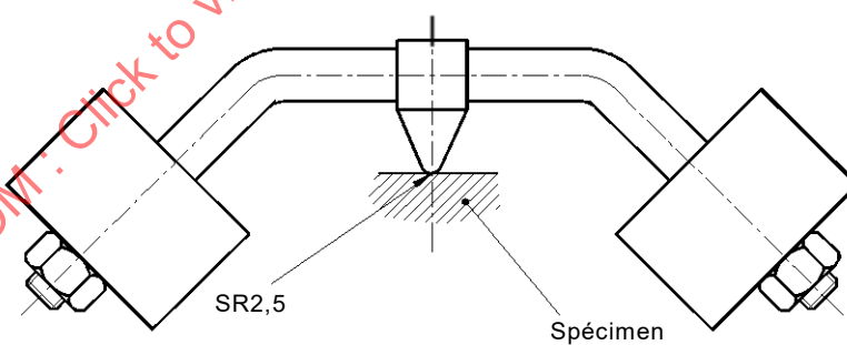
Figure 9 – Appareil pour la résistance à la compression
