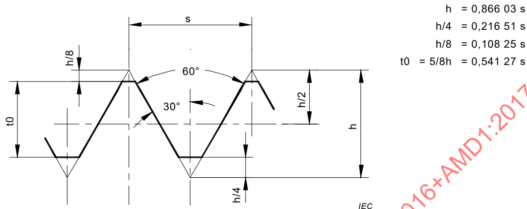
Profil de base a
