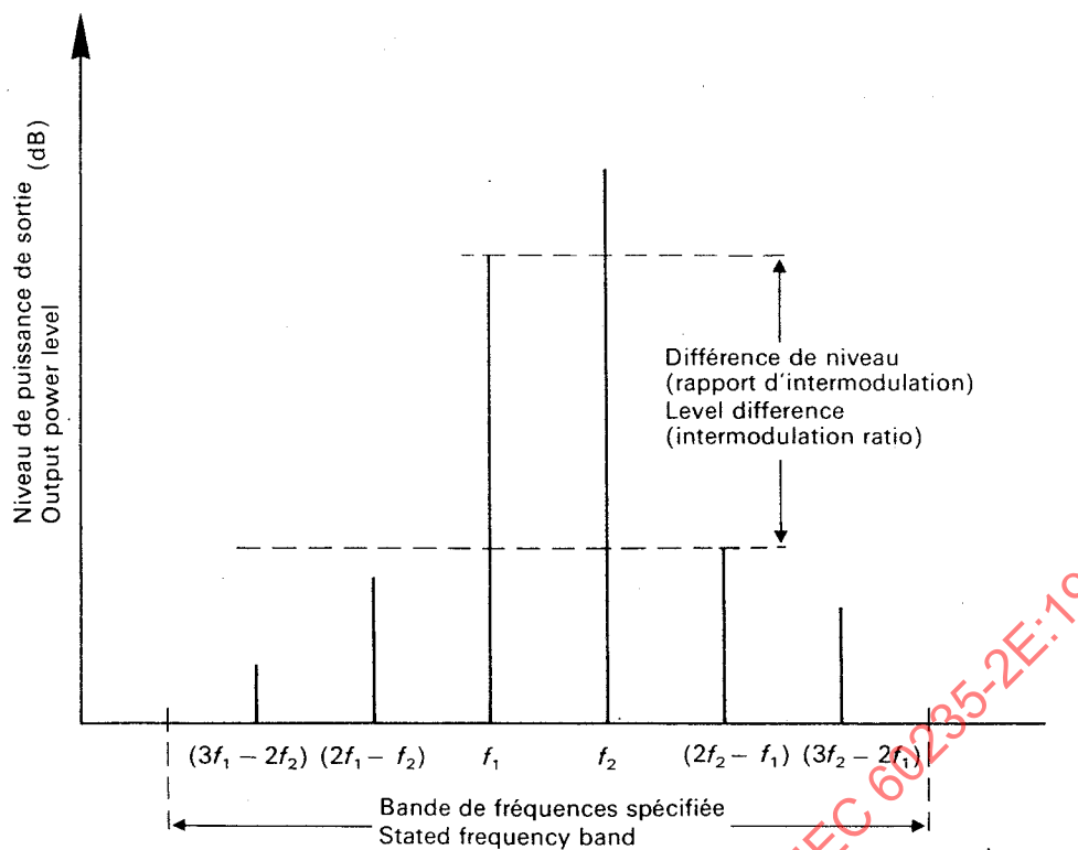
FIG. 53. — Intermodulation: méthode à deux fréquences. Intermodulation: two-frequency method.
